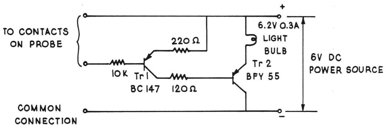
Fig. III-4: Basic Amplifier Unit
